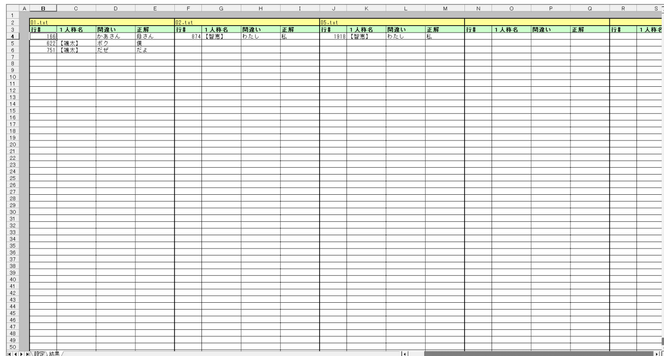
図2. 結果表示
