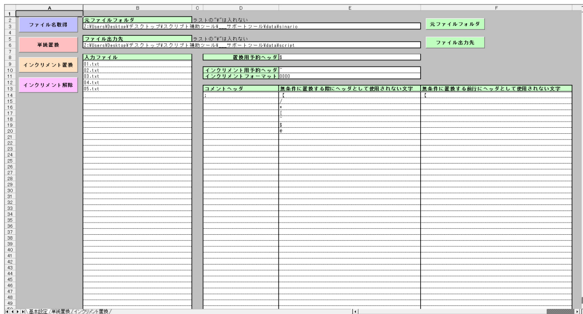
図1. 設定画面
