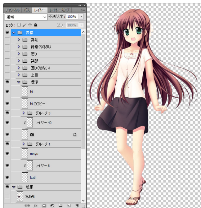
図2. 読込 PSD
