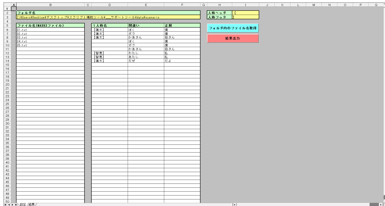
図1. 設定画面
